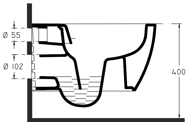
Seitenansicht
