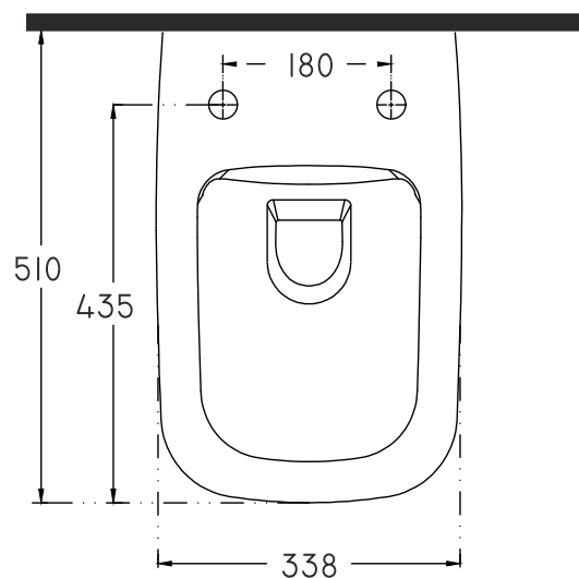
Wandanschluss
