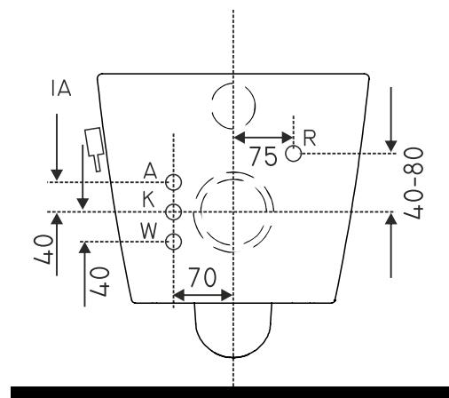
Wandanschluss
