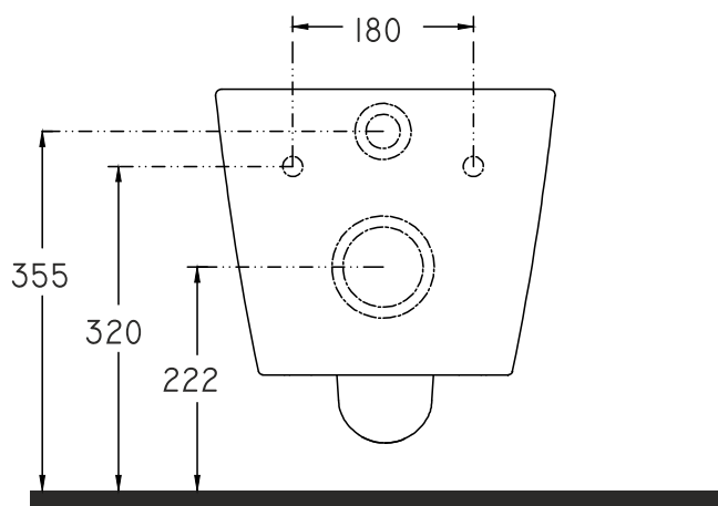
Frontansicht
