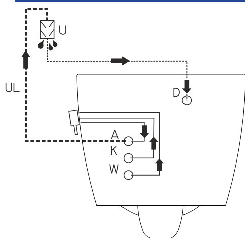
A Anschluss mit Kalt-Warmwasser und Rohrunterbrecher
