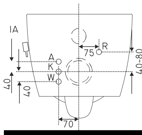
Wandanschluss
