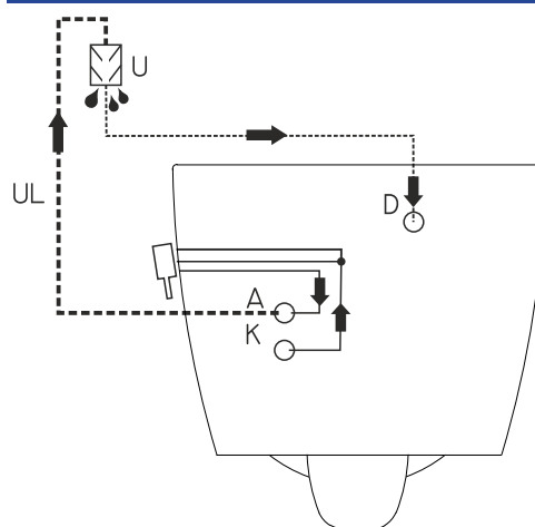
B Anschluss mit Kaltwasser und Rohrunterbrecher
