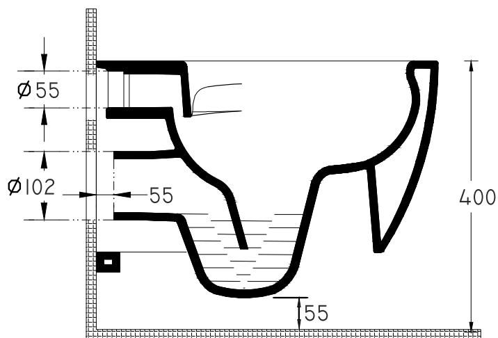
Seitenansicht
