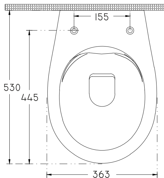
Wandanschluss
