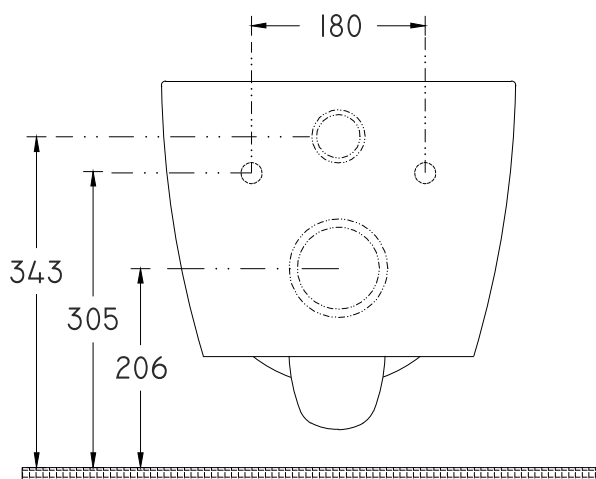
Frontansicht
